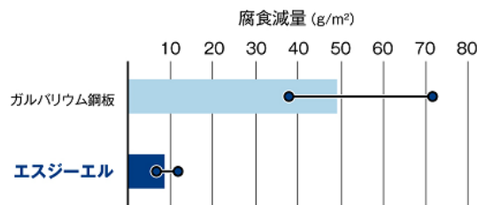
複合サイクル試験による腐食減量 0.5%NaCl-JASO/180C
